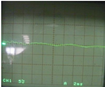
Gambar 16. Gelombang Hasil Pengujian dengan Beban 3,3 kΩ
